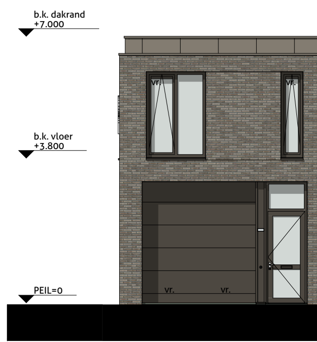
Voorgevel 1:100
