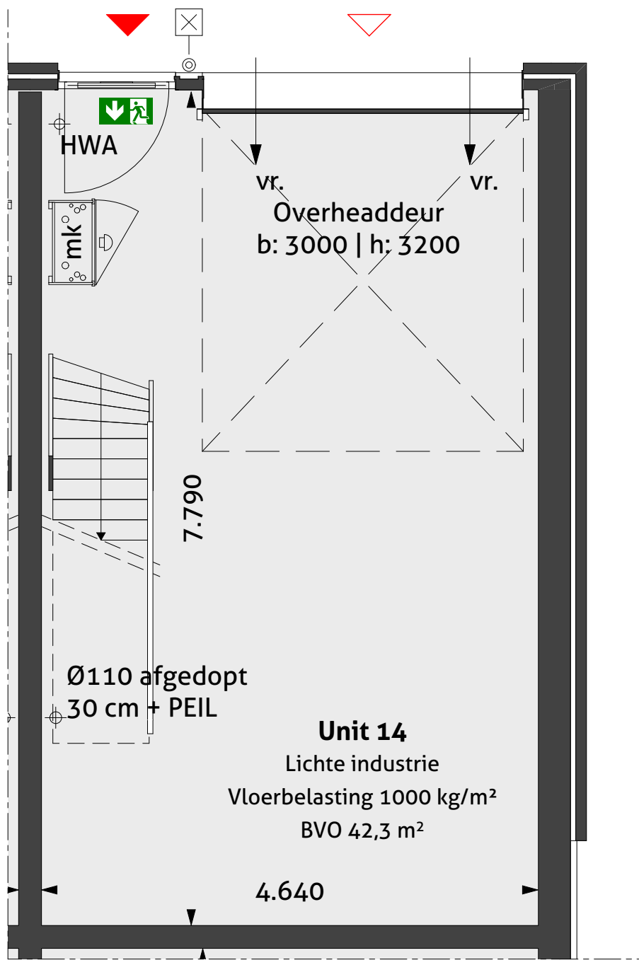
Begane grond 1:50
