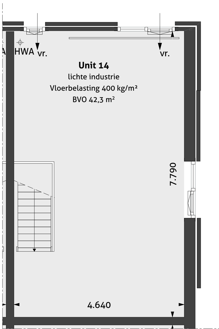
Verdieping 1:50
