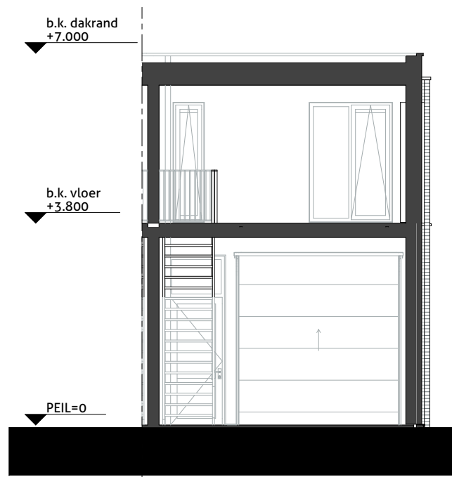
Doorsnede 1:100
