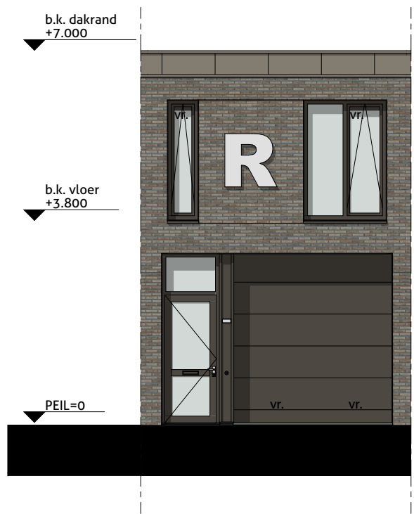
Voorgevel 1:100
