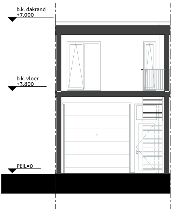
Doorsnede 1:100
