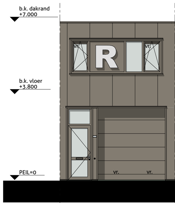
Voorgevel 1:100
