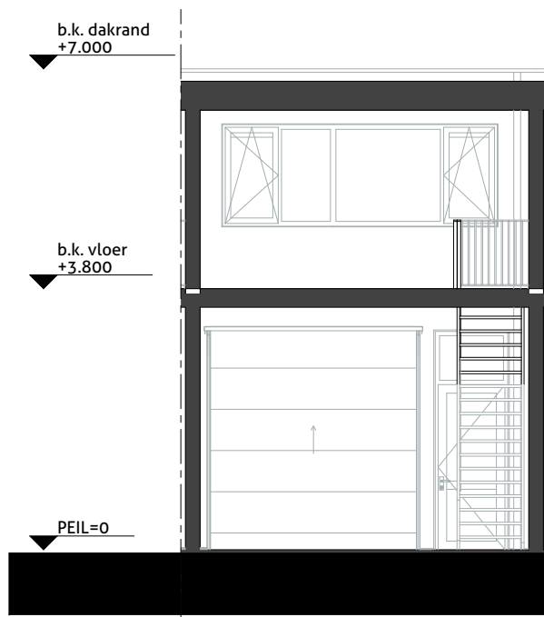
Doorsnede 1:100
