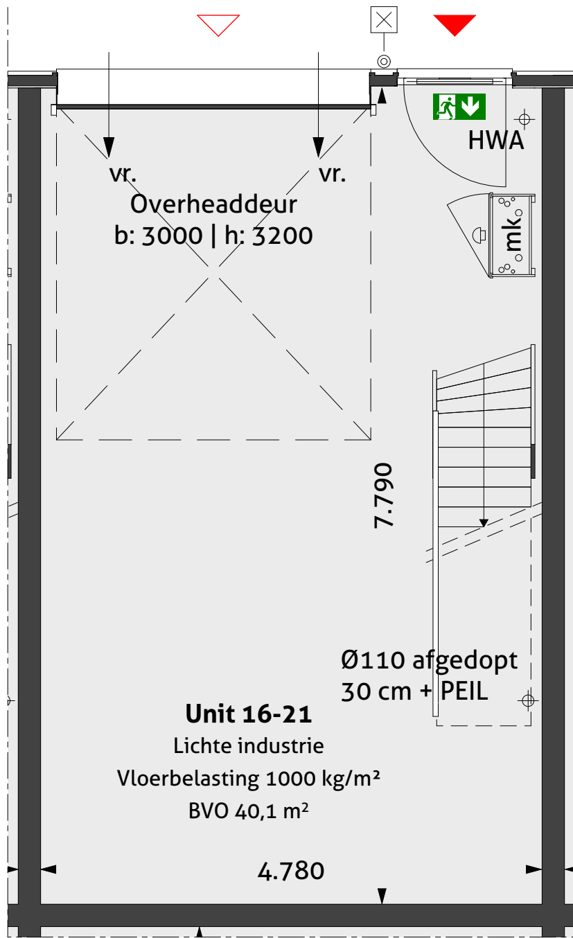
Begane grond 1:50
