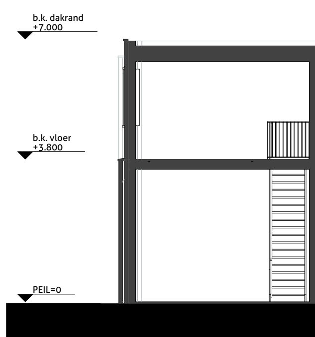
Doorsnede 1:100
