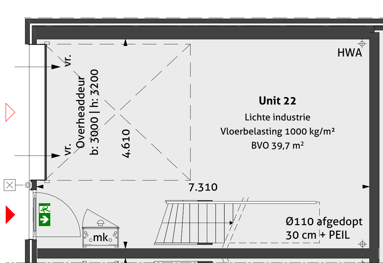
Begane grond 1:50
