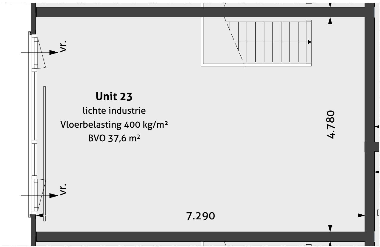
Verdieping 1:100
