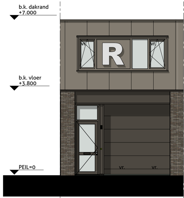
Voorgevel 1:100
