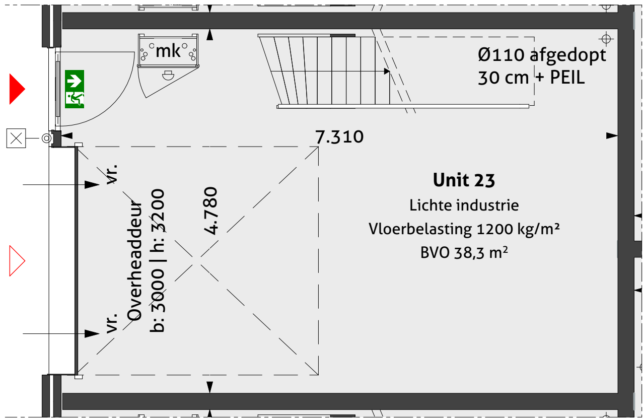
Begane grond 1:100
