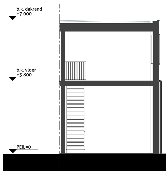
Doorsnede 1:100
