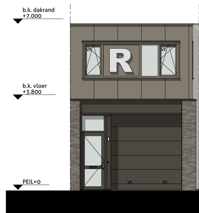
Voorgevel 1:100
