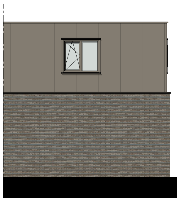
Zijgevel 1:100
