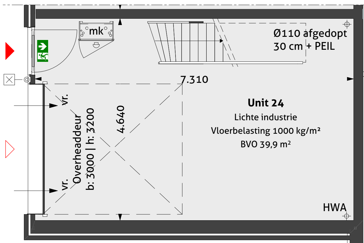
Begane grond 1:100
