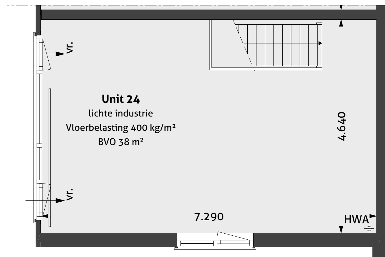
Verdieping 1:100
