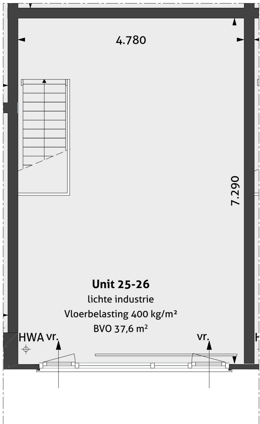
Verdieping 1:50
