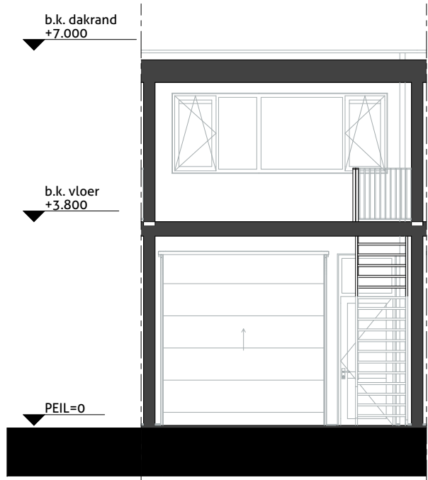
Doorsnede 1:100
