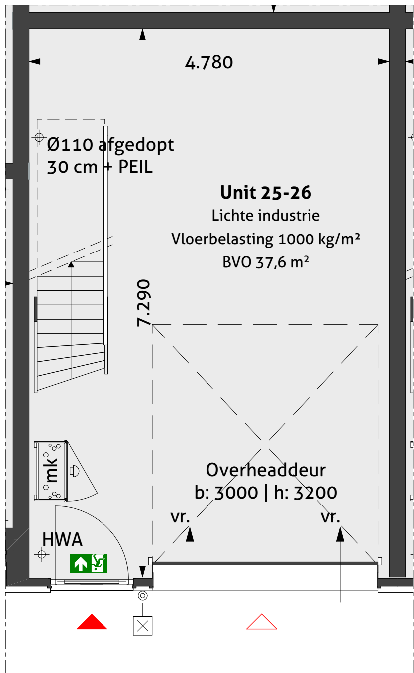
Begane grond 1:50
