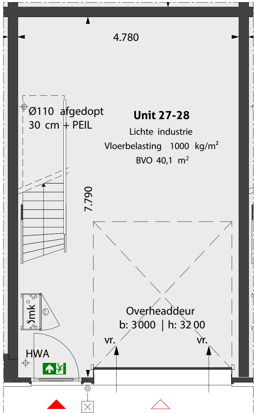
Begane grond 1:50
